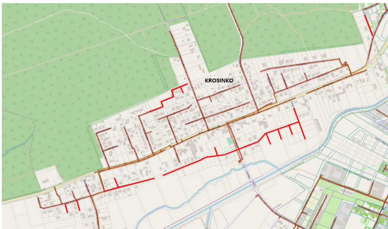
Krosinko – kanalizacja sanitarna — Istniejąca sieć kanalizacji sanitarnej — Projektowana sieć kanalizacji sanitarnej
