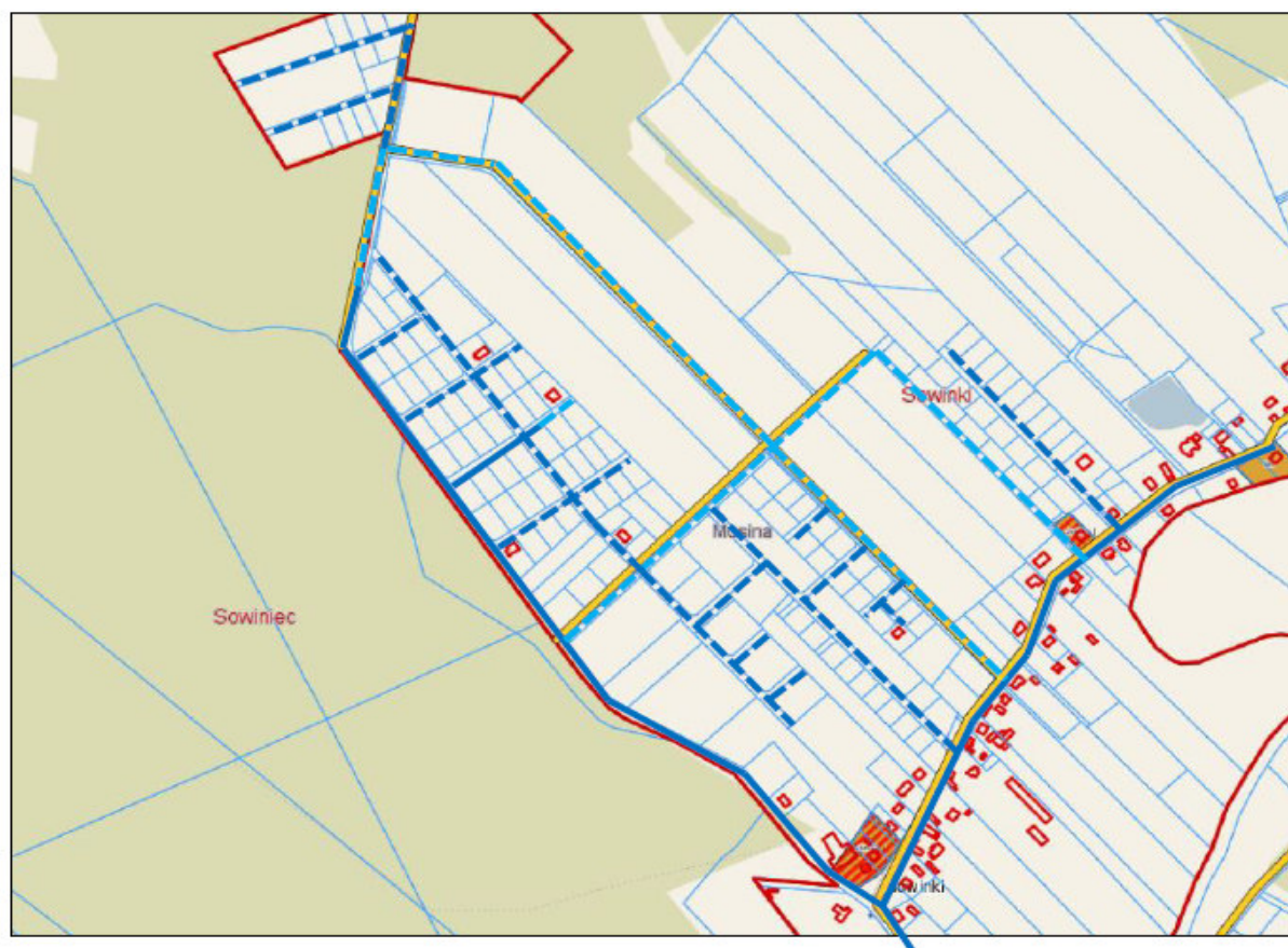
3-03-17-149-1 - Mosina - sieć wodociągowa w m. Sowinki
