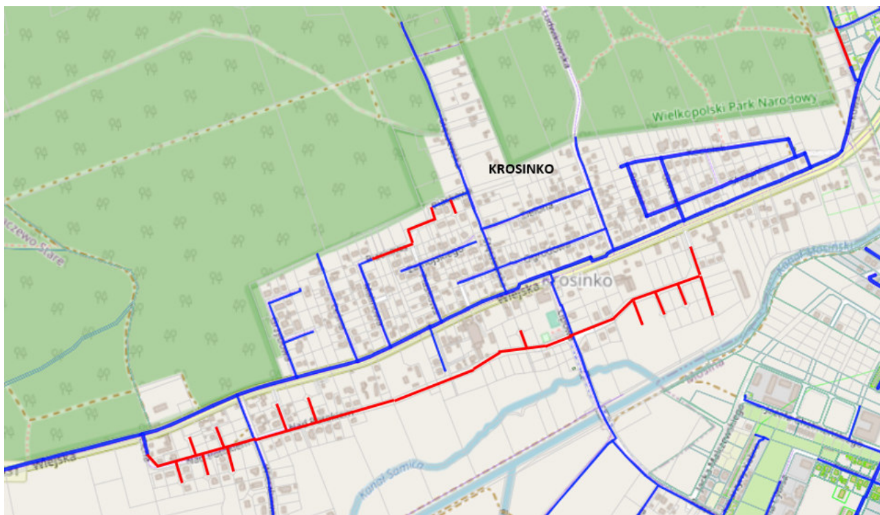
Krosinko – sieć wodociągowa
