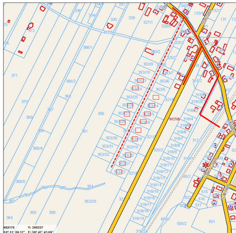
5-03-20-128-1 Pecna, ul. Topolowa Kanalizacja sanitarna istniejąca Ks. Projektowana : przewód grawitacyjny DN200mm, L = 460m
